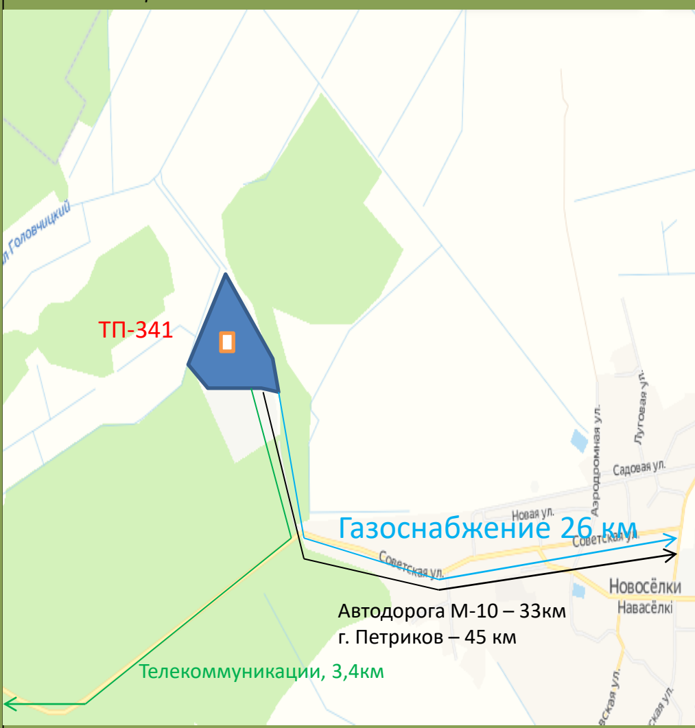
Схема площадки
